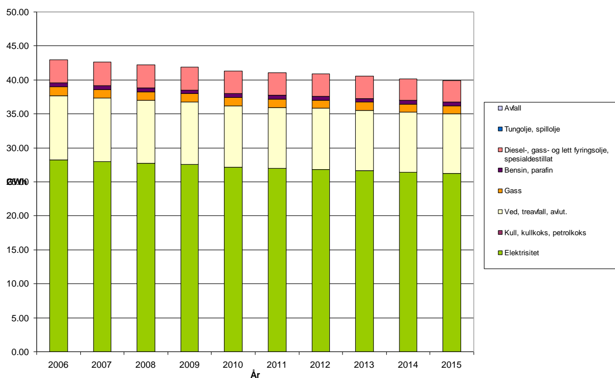
Figur 4.4 Energiprognose Rendalen Kommune 2006-2015
