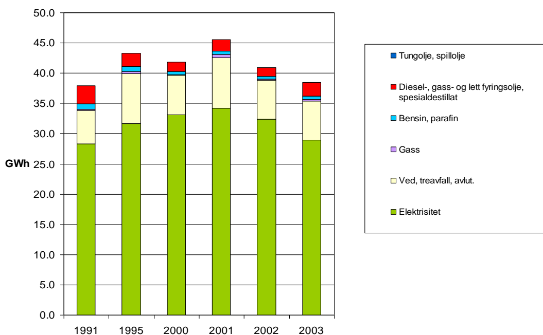
Figur 4.3 Oversikt energibruk Folldal Kommune 1991, 1995 og 2000 - 2003
