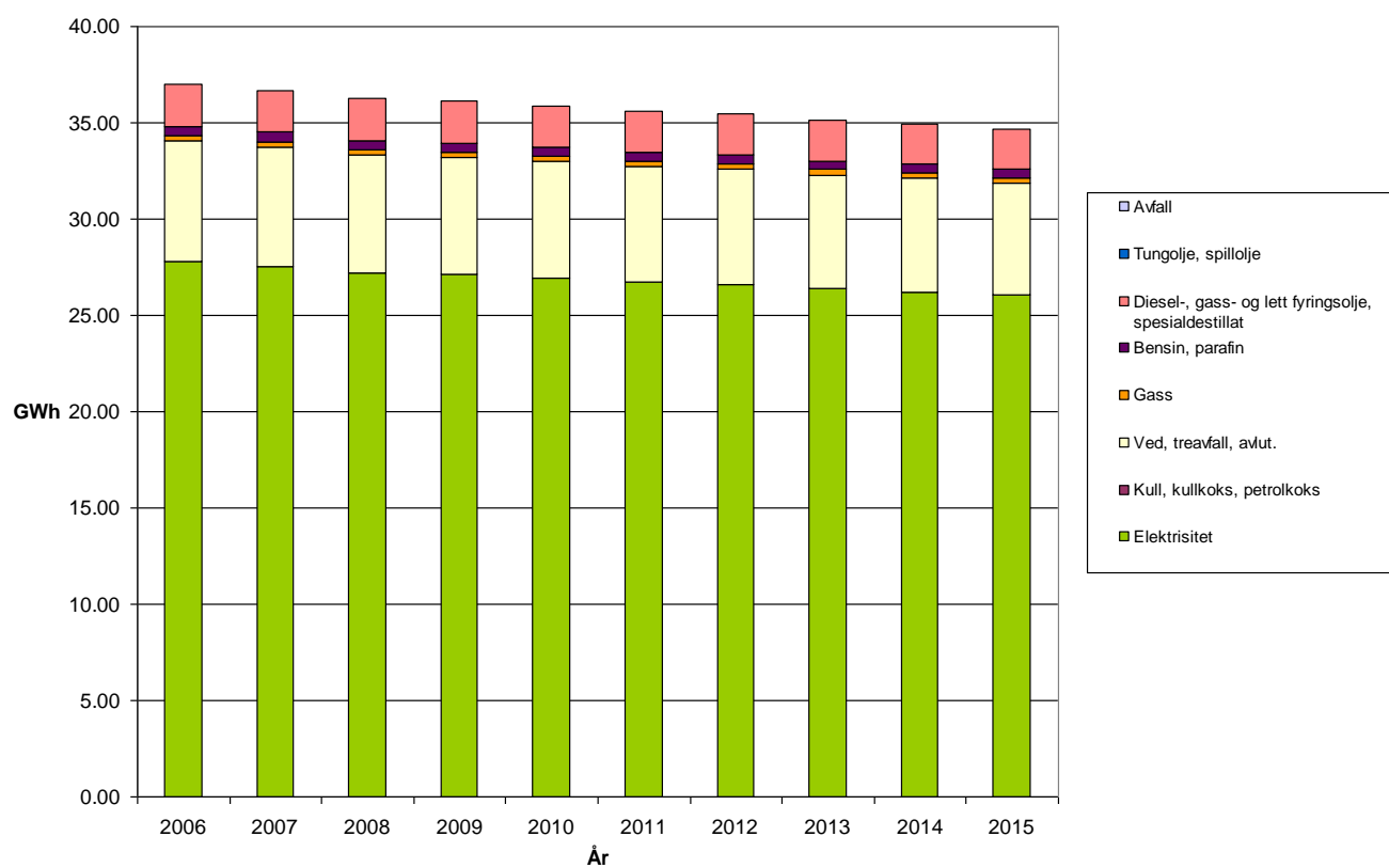
Figur 4.4 Energiprognose Folldal Kommune 2006 - 2015
